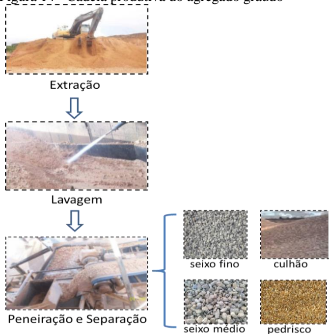
Figura 14 - Cadeia produtiva do agregado graúdo
