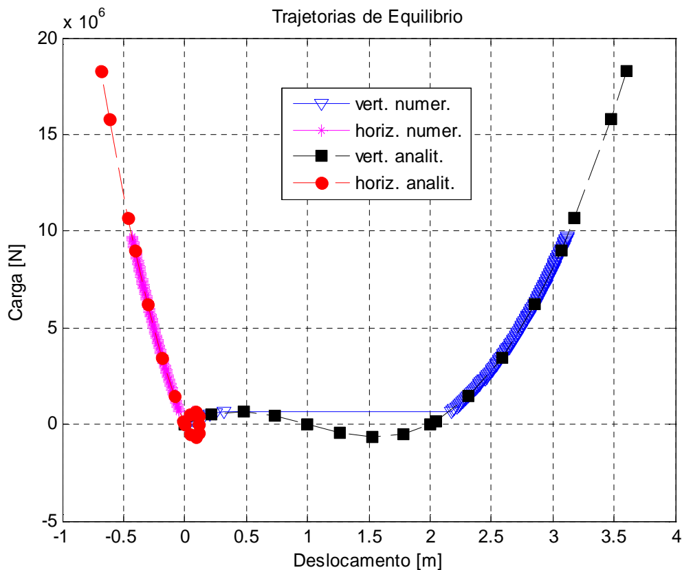
Figura 6.11. Trajetória de Equilíbrio da Estrutura
